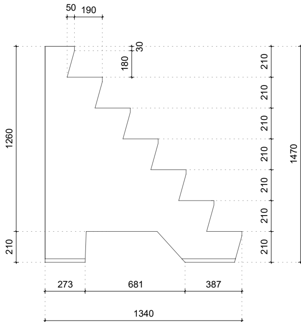
Zijaanzicht
