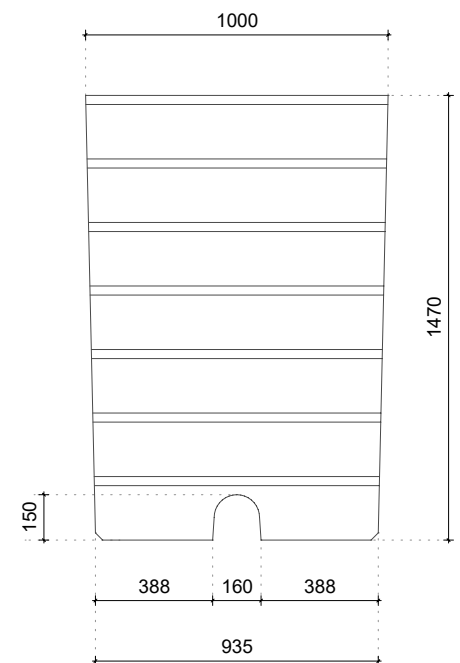
Vooraanzicht
